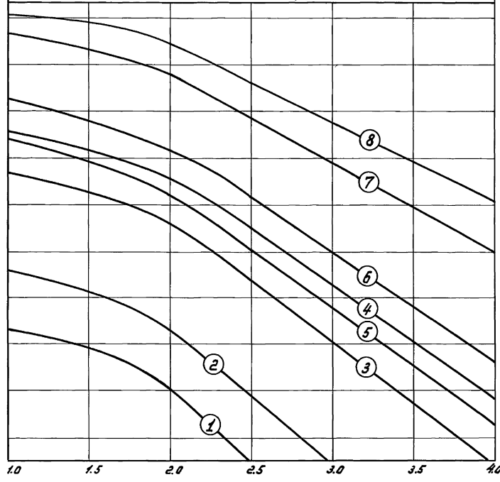
Основное сочетание нагрузок
